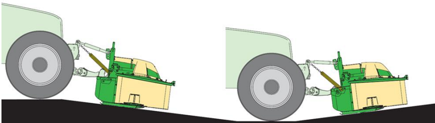
Prevedenie Pull – ťahaná verzia, hydropneumatické nastavenie prítlaku lišty-sériovo
